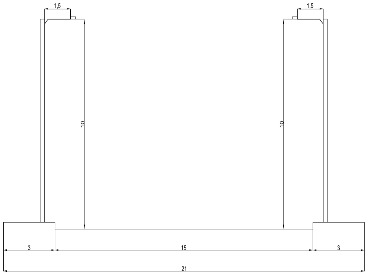
PERFIL 5 VIA V4-V5
