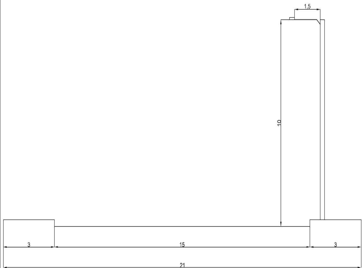
PERFIL 3 VIA V4-V5
