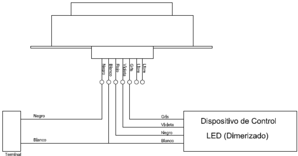
Ilustración 1 : Conexión de receptáculo de fotocontrol
