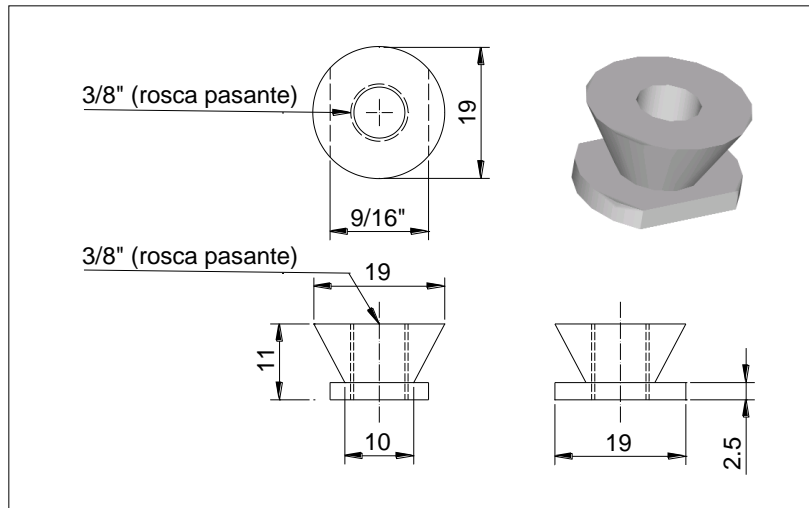
Ilustración 2 : Detalle de tuerca cónica
