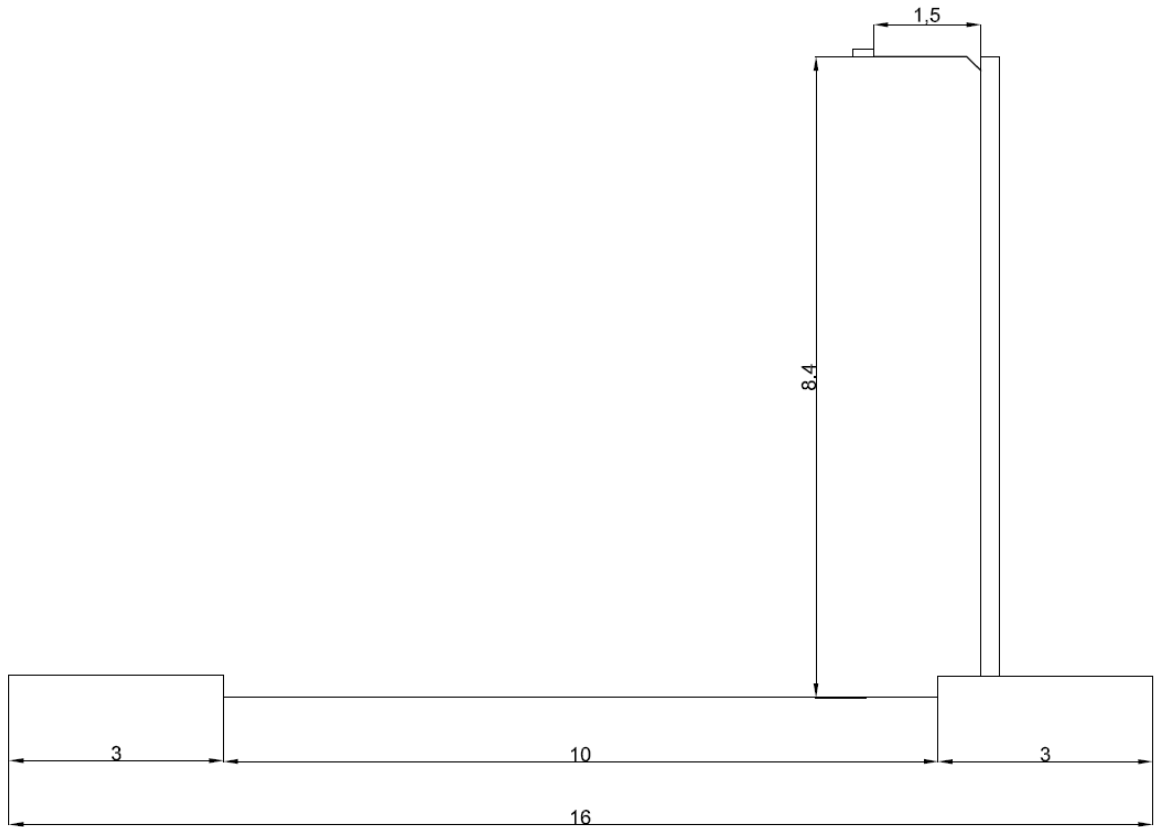
PERFIL 2 VIA V6
